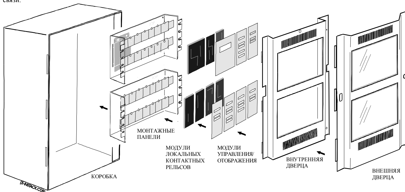
Рис. 1. компоненты системы EST3
