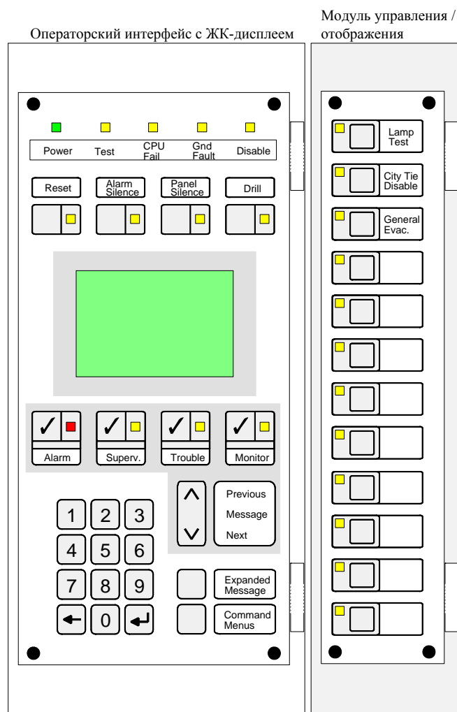
Рис. 2. Дополнительный модуль операторского интерфейса и модуль управления/отображения
